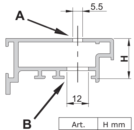
SEZ. C-C
