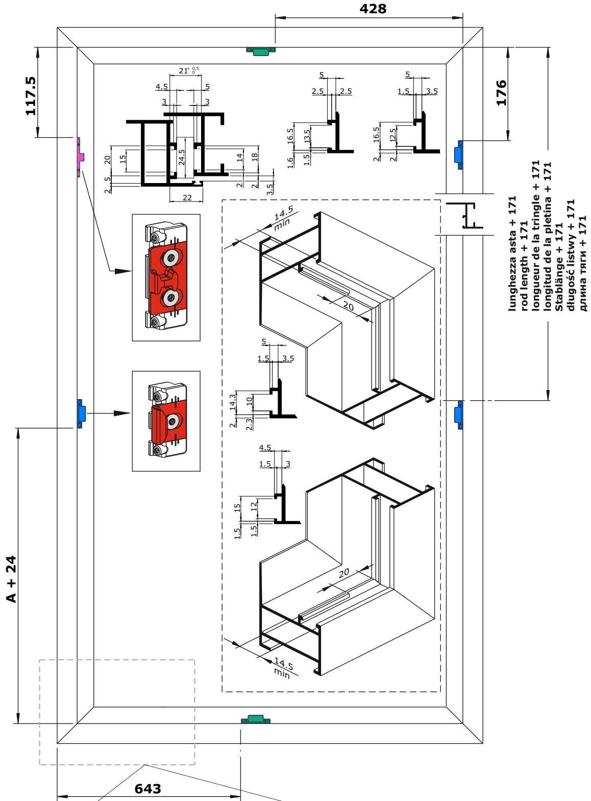
3201.20R - 3201.20L Con fulcro verticale laterale - With lateral vertical fulcrum Avec dispositif de verrouillage vertical latéral Con fulcro vertical lateral - Mit senkrechtem Drehpunkt z podparciem obrotowym pionowym С вертикальным шпингалетом
