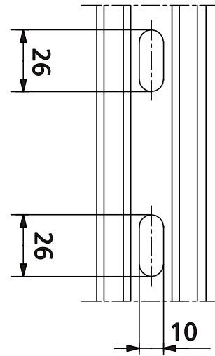
Lavoraz. per pacchi di movimentazione
