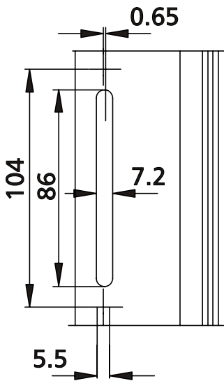
Lavorazione per innesti
