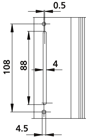
Lavoraz. per pacchi di movimentazione
